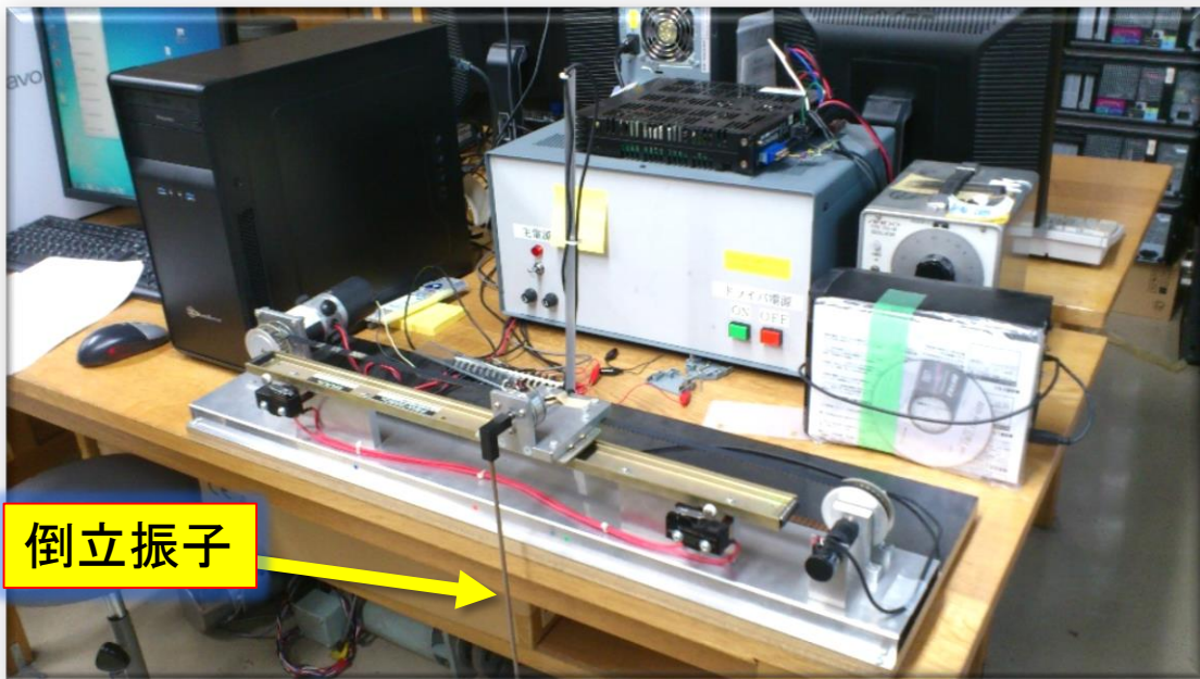
倒立振り子
