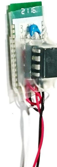
実装 3.3Vレギュレータ, キャパシタ込々
