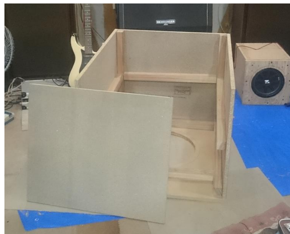
補強(MDF20mmは薄い!)
